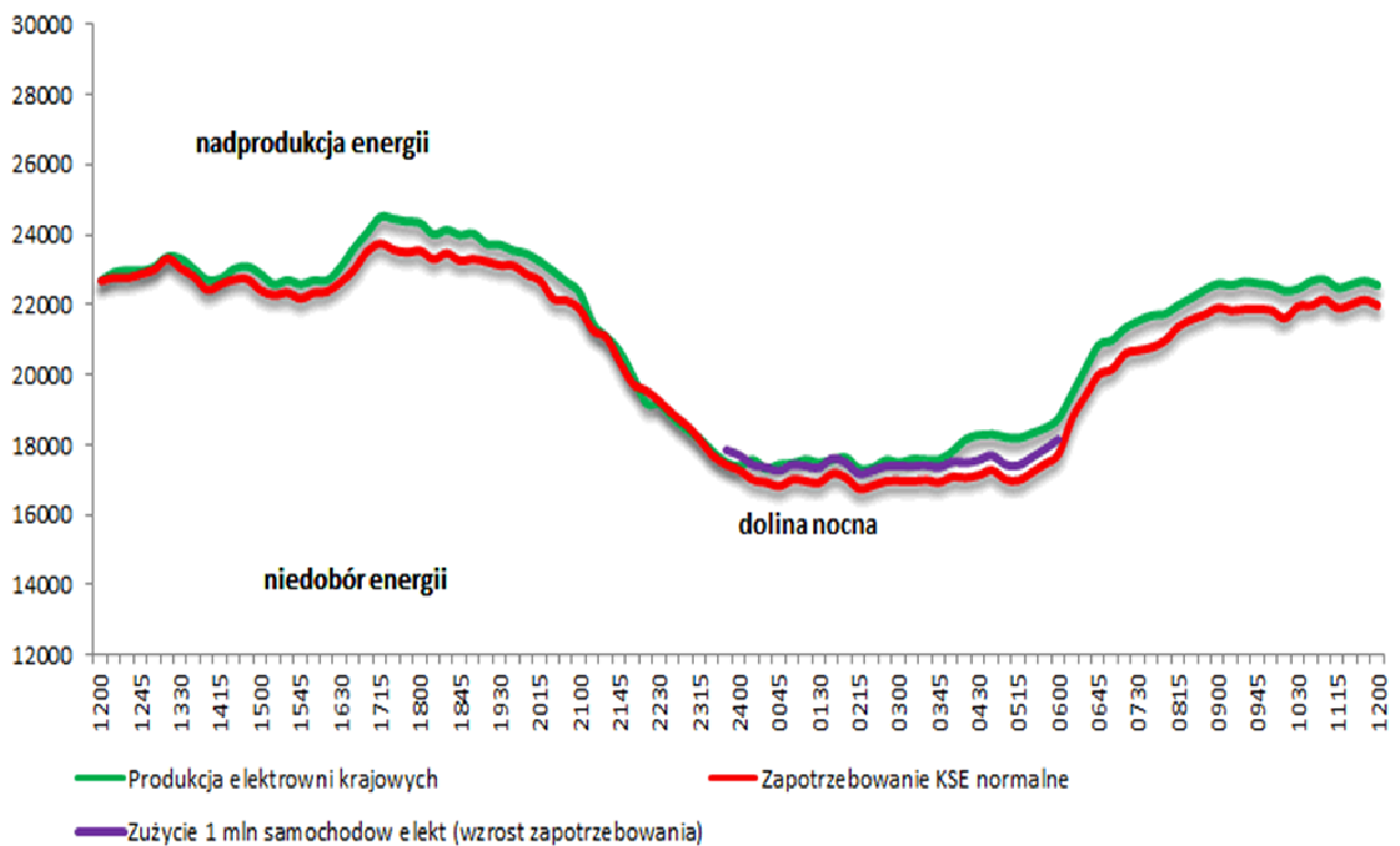
Wykres nr 1 Zapotrzebowanie KSE (Krajowej Sieci Energetycznej) i produkcja elektrowni krajowych.
